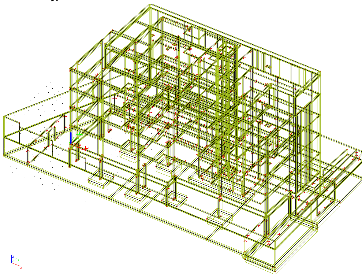
3D výpočetní model- axonometrie celku
