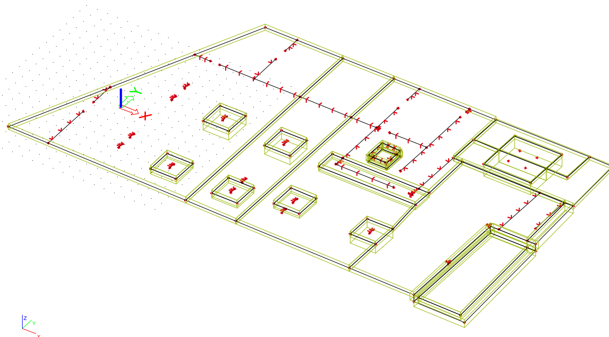
3D výpočetní model- axonometrie základové desky
